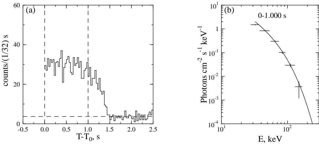
Fig. 2.7.— Burst 820102.
