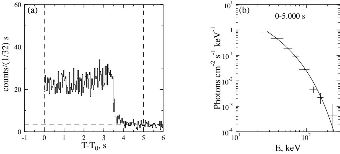
Fig. 2.6.— Burst 811201.
