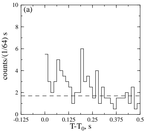
Fig. 2.8.— Burst 820215.
