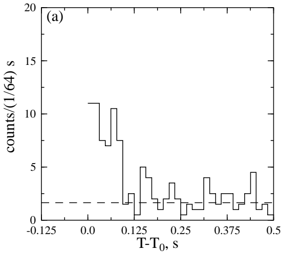
Fig. 2.10.— Burst 820423a.
