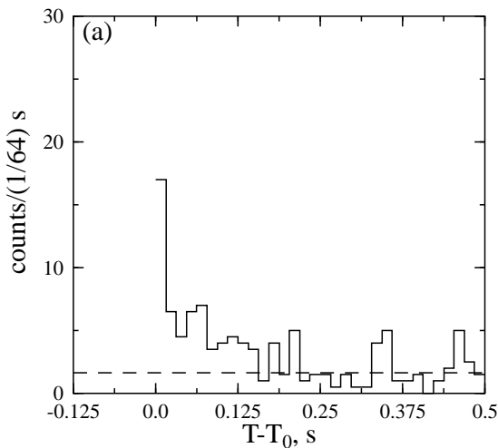
Fig. 2.12.— Burst 820510.
