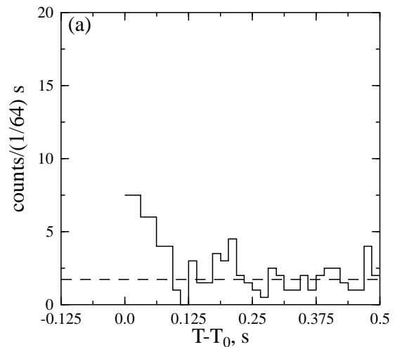
Fig. 2.13.— Burst 820530.
