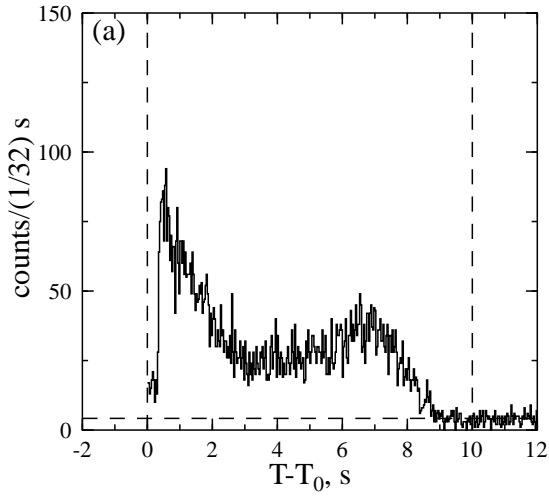
Fig. 2.9.— Burst 820227.
