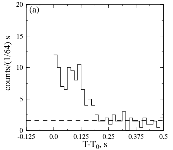
Fig. 2.11.— Burst 820423b.
