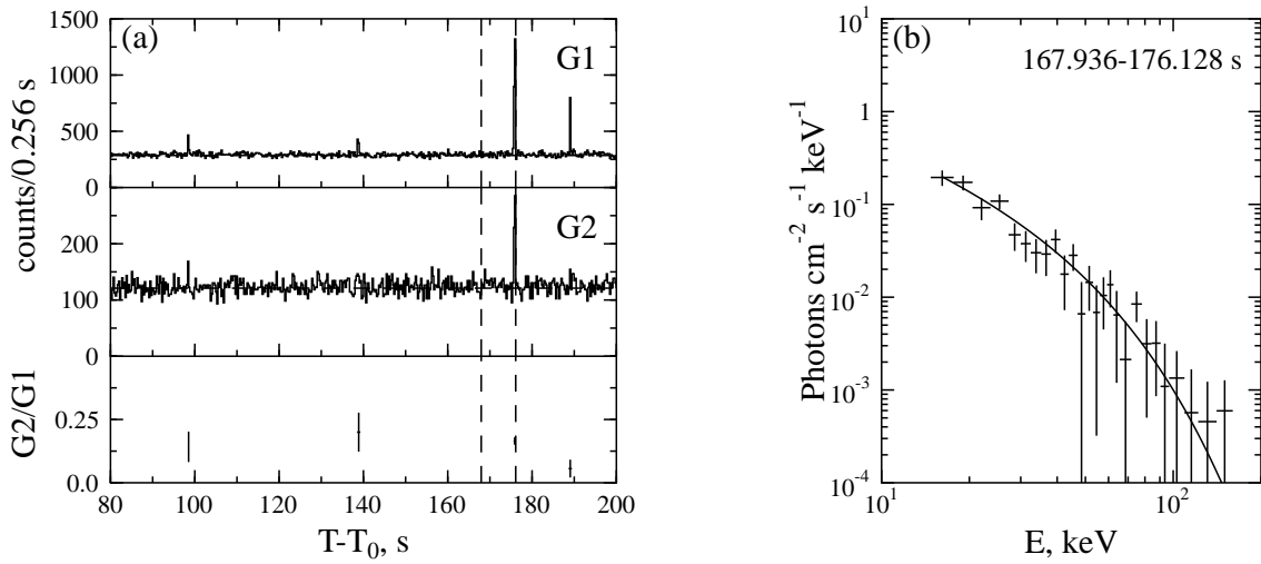
Fig. 3.14.— Burst 980530a (continued).
