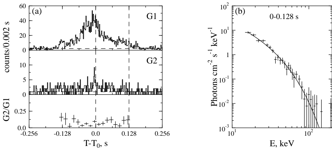
Fig. 3.16.— Burst 980530b.
