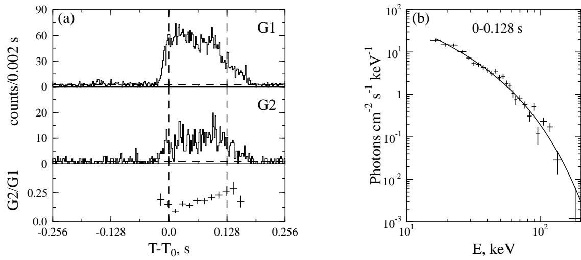
Fig. 3.26.— Burst 980821.
