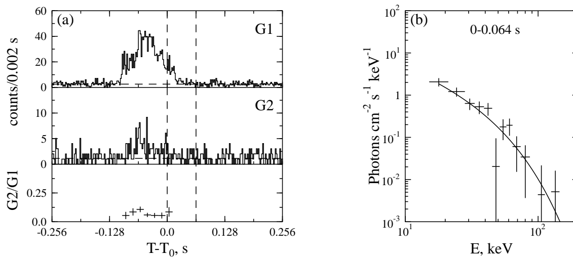
Fig. 3.36.— Burst 980831a.
