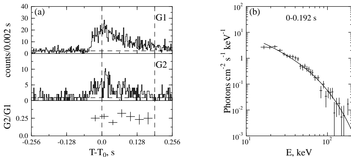
Fig. 3.50.— Burst 980927.
