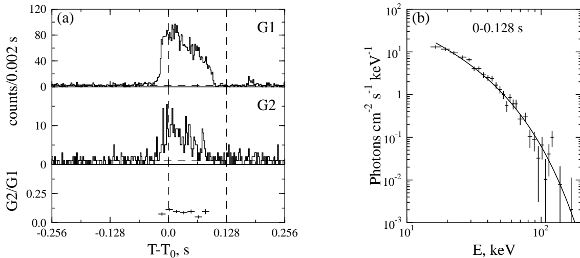
Fig. 3.49.— Burst 980917.
