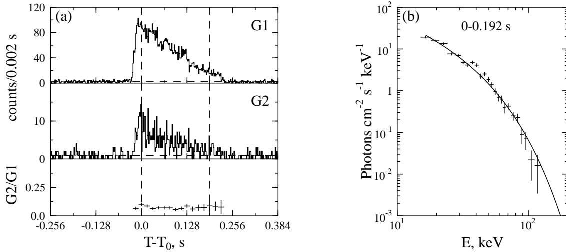
Fig. 3.48.— Burst 980915a.
