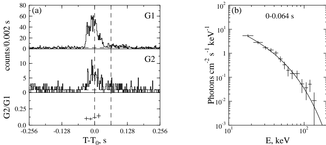
Fig. 3.59.— Burst 981028a.
