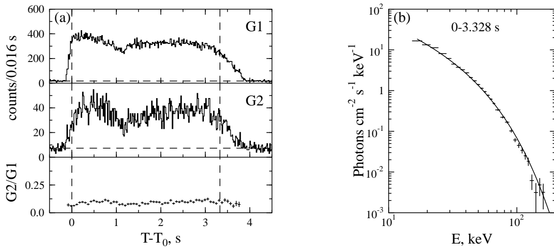
Fig. 3.60.— Long burst 981028b.
