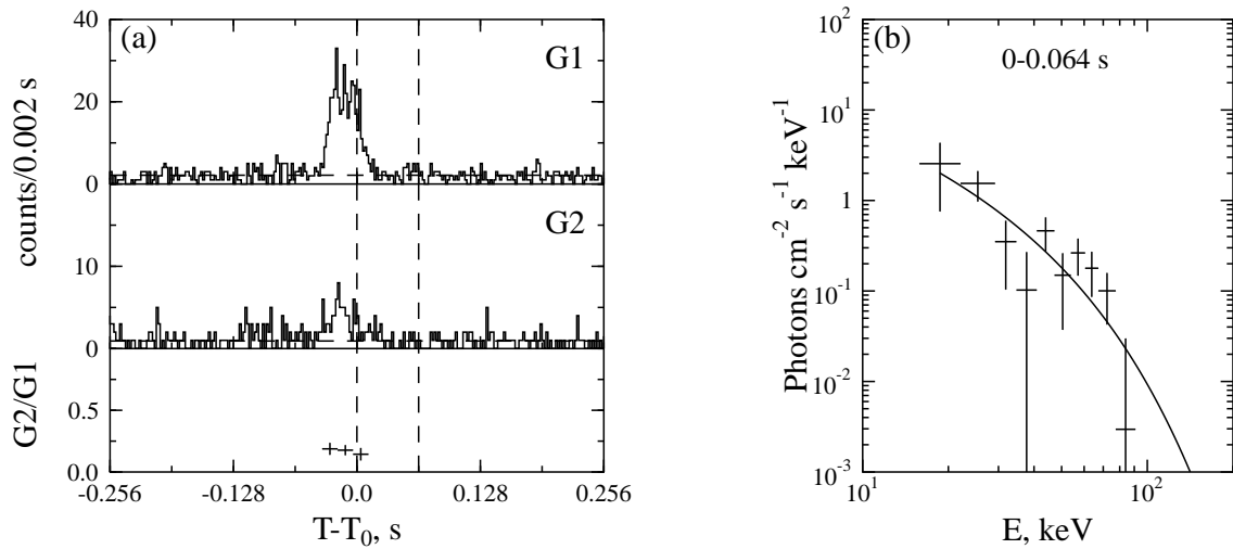
Fig. 4.17.— Burst 990104.
