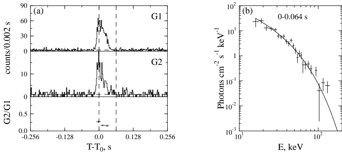
Fig. 4.18.— Burst 990125.
